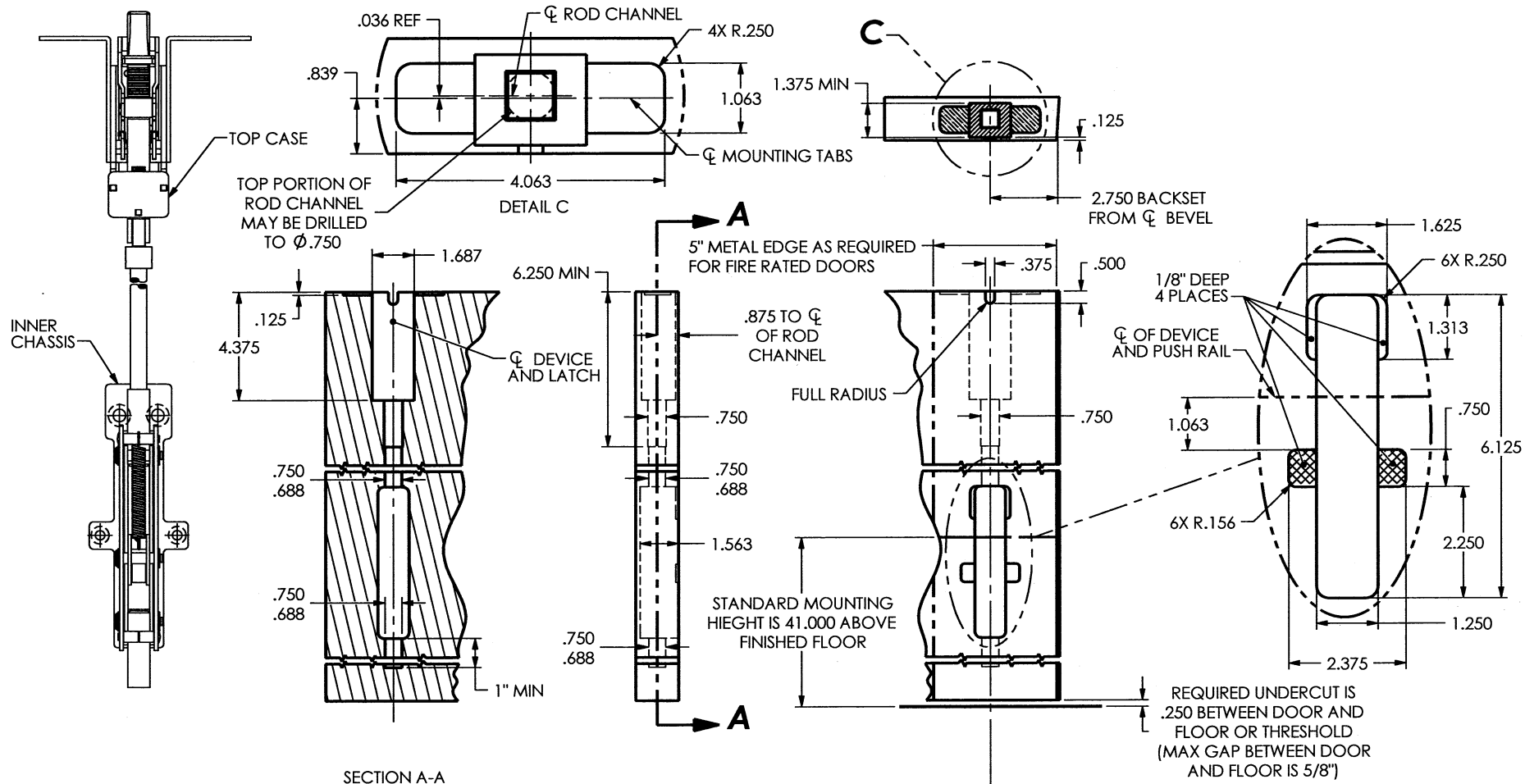
SECTION A-A
